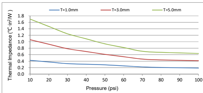
Thermal Impedance
