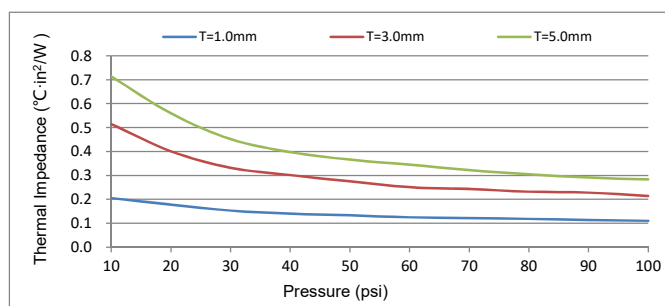
Thermal Impedance
