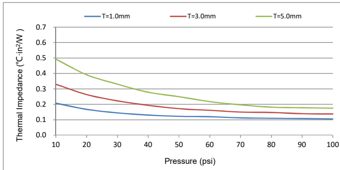
Thermal Impedance
