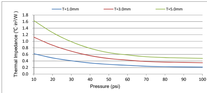
Thermal Impedance
