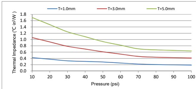
Thermal Impedance
