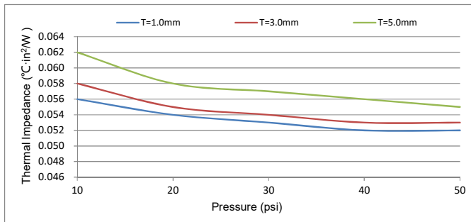
Thermal Impedance
